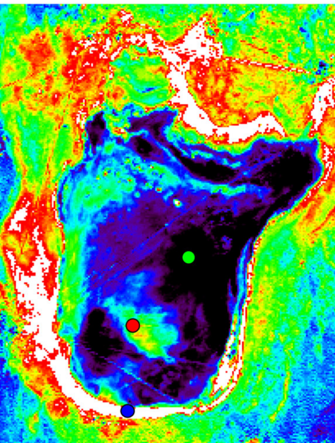
OLI - SSSI
