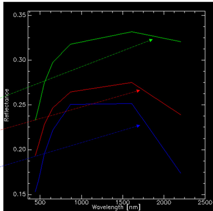
OLI - spectra
