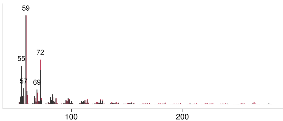
9-Octadecenamide
