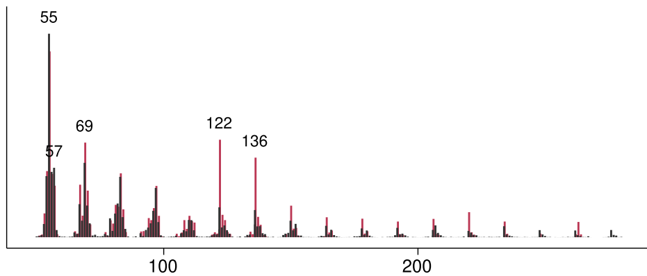
Oleonitrile
