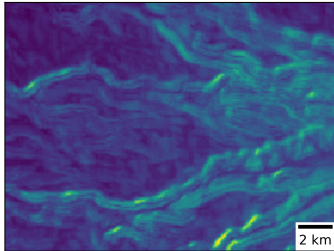
(b) CNN
